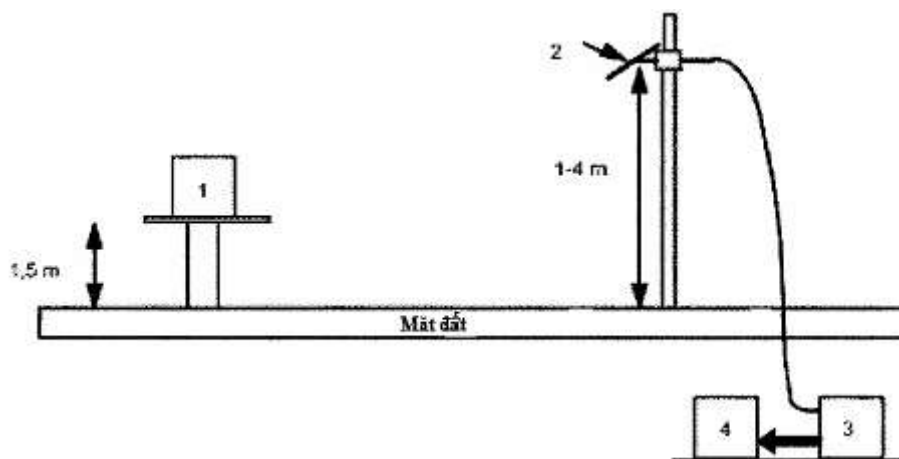
Hình C.1 - Vị trí đo ngoài trời
